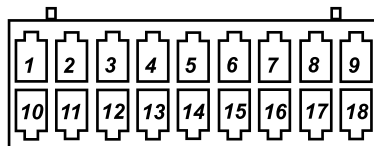
Вид со стороны проводов Рис. 4
