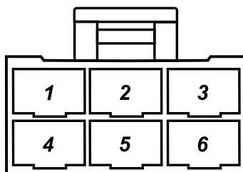
Вид со стороны проводов Рис. 8
