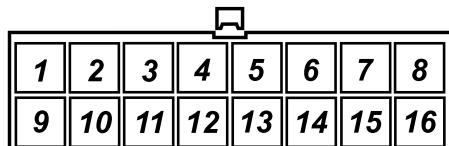
Вид со стороны проводов
