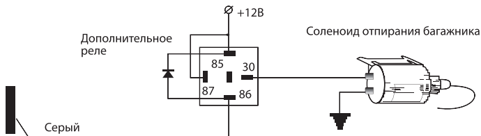
Рис.2.2. Подключение электропривода отпирания багажника.
