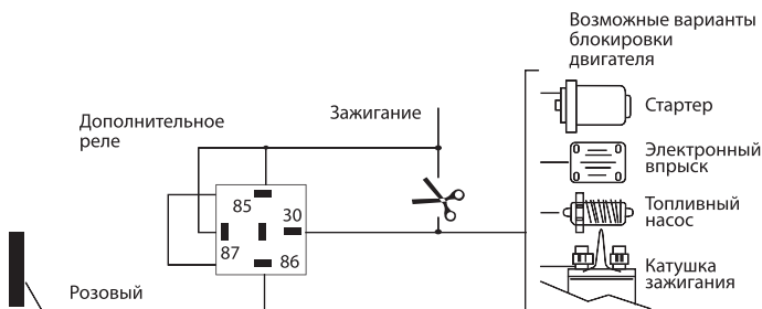
Рис.2.3. Схема организации дополнительной блокировки двигателя.
