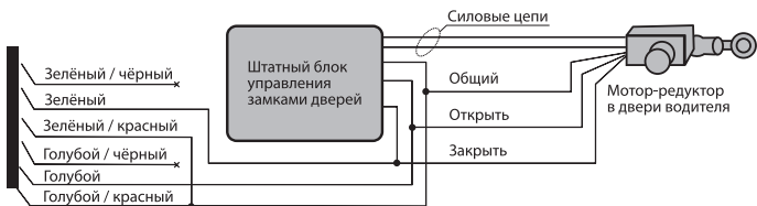
Рис.2.5. Установка новых электроприводов замков дверей.
