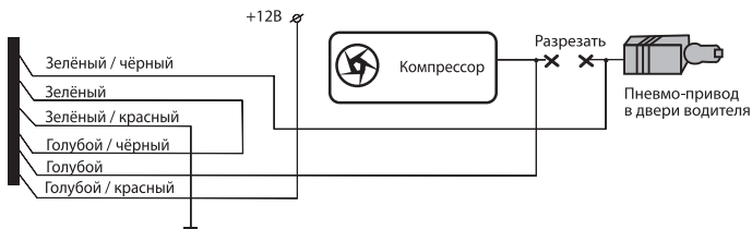
Рис.2.7. Подключение к штатной системе управления пневдоприводами замков дверей. Перемычка J1 в центральном блоке должна быть удалена.
