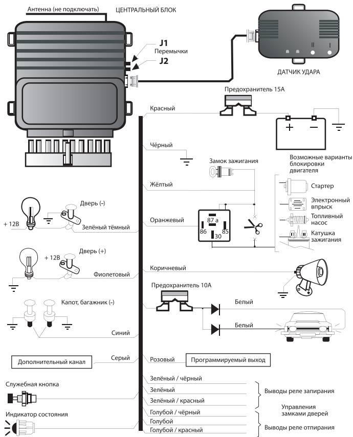
Рис.2.1. Схема подключения сигнализации PHANTOM Voyager.
