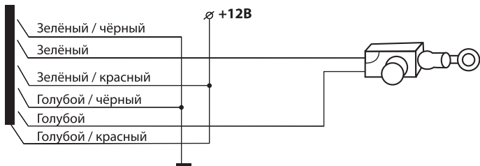
Рис.2.5. Установка новых электроприводов замков дверей.
