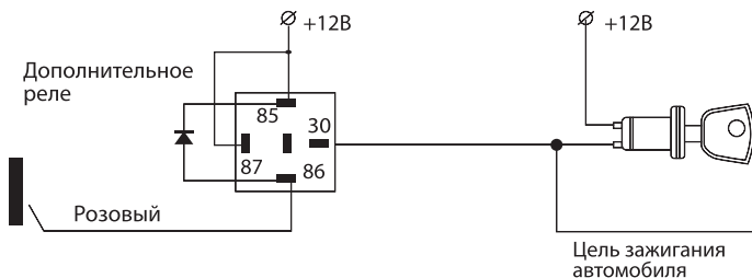
Рис.2.4. Схема организации поддержки зажигания.
