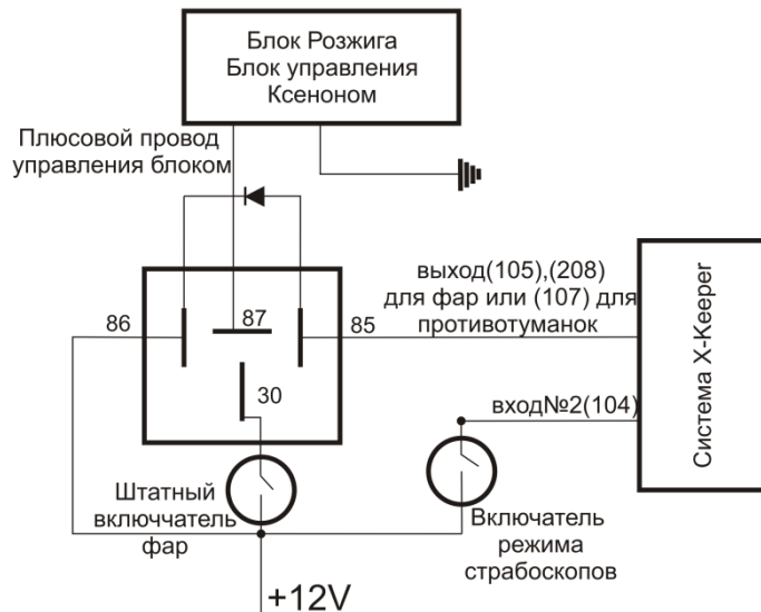
Схема подключения №1
