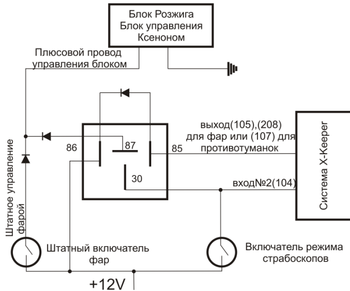
Схема подключения №2
