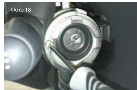
Фото 18 3.15. В резьбовое отверстие корпуса «Защиты корпуса» закрутите винт М5 до упора резьбы, предварительно нанесите анаэробный герметик (типа Loctite 243). (Фото №18)
