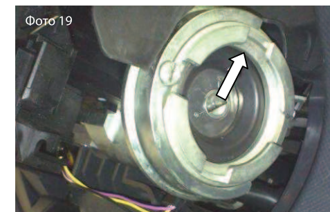
Фото 19 3.16. Приподнимите «Защиту корпуса» в верх и подтяните винт М5 на хомуте, для фиксации изделия в данном положении (Фото №19).
