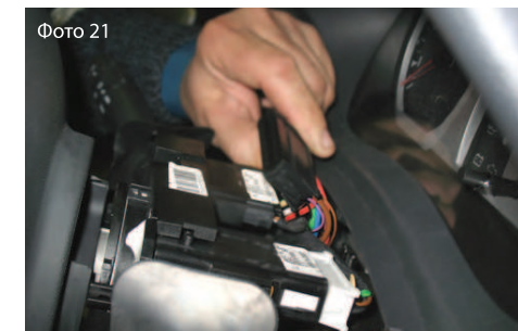
Фото 21 3.18. Подключите разъем проводов переключателя поворотов (Фото №21).
