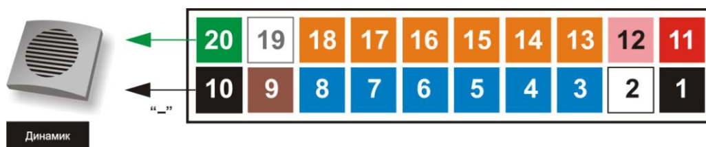
Рис. 7 Схема подключения внешнего акустического устройства
