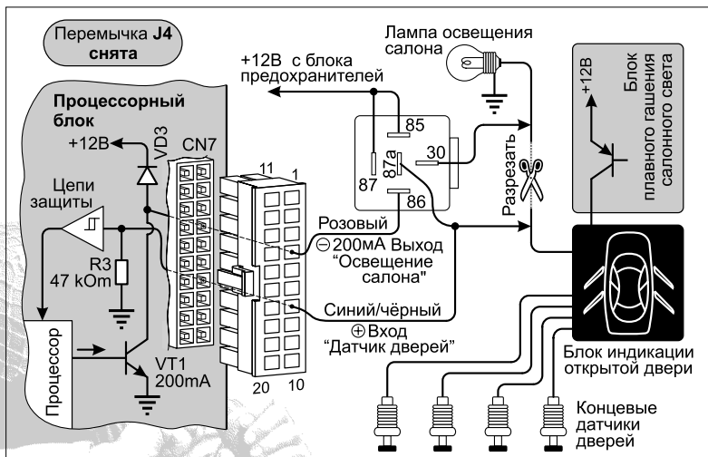
Рис. 15. Подключение входа датчиков дверей и выхода управления освещением салона. Для автомобилей, в которых включение освещения салона производится при подаче +12В. Быстрое гашение освещения салона после того, как он был включен системой PARTISAN RX-5. Использована функция учета задержки выключения света в салоне – джампер J4 снят.
