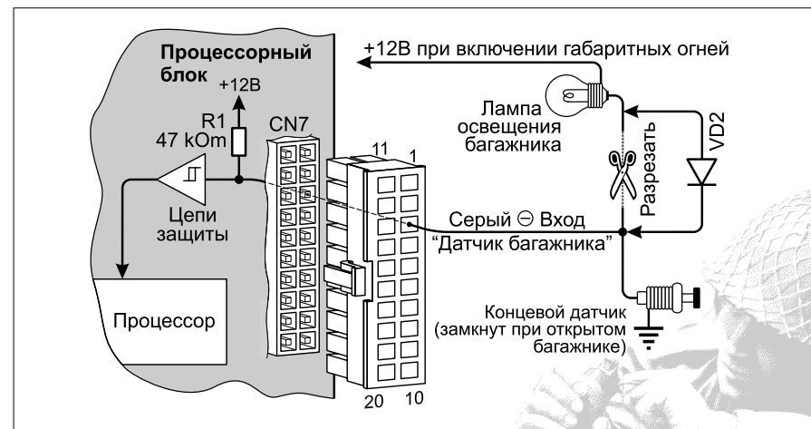
Рис. 9. Подключение концевого датчика открытия багажника. Для автомобилей, в которых этот датчик использован для включения лампы освещения багажника. Питание на лампу подается при включении габаритных огней. Датчик соединяет выходной провод с массой при открытом багажнике.
