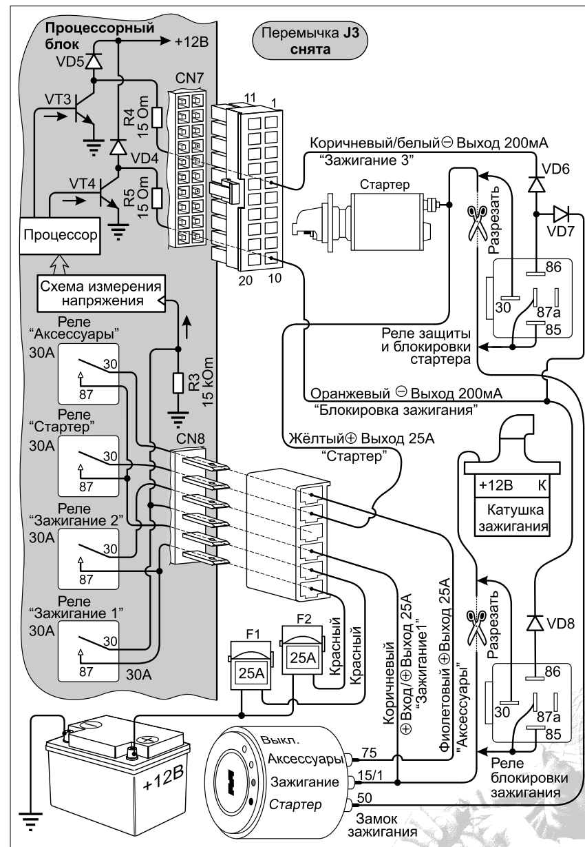
Рис. 19. Схема подключения нормально-замкнутого реле блокировки зажигания и реле защиты и блокировки стартера.
