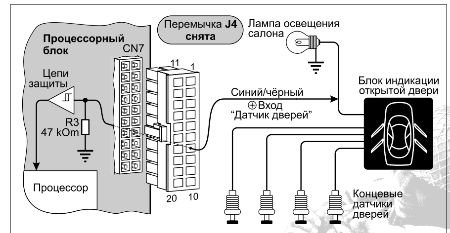
Рис. 17. Подключение входа датчиков дверей. Для автомобилей, в которых включение освещения салона производится при подаче +12В. Выход управления освещением салона не используется. Использована функция учета задержки выключения света в салоне – джампер J4 снят.
