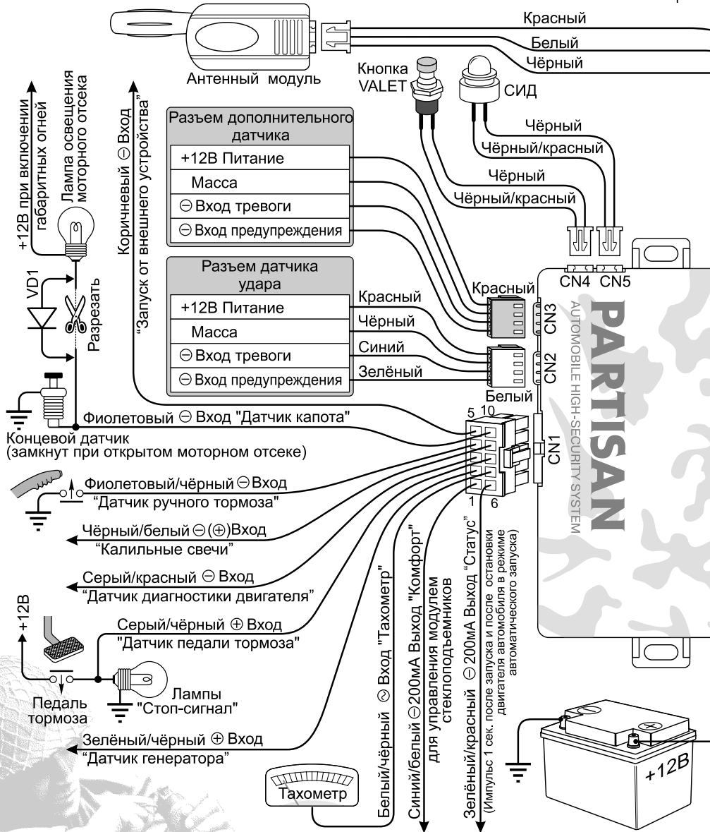
Рис. 1. Схема подключения PARTISAN RX-5
