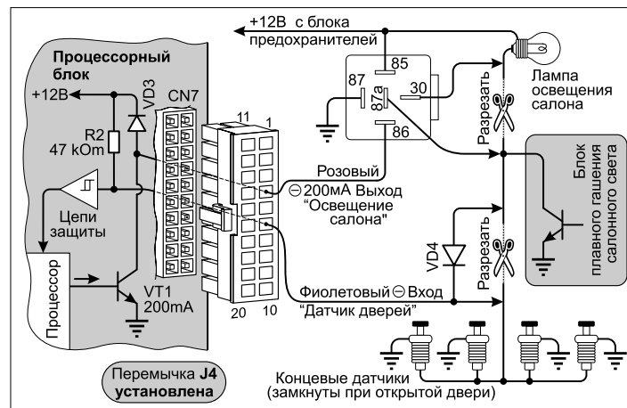
Рис.12. Подключение входа датчиков дверей и выхода управления освещением салона. Для автомобилей, в которых включение освещения салона производится при подаче массы. Быстрое гашение освещения салона после того, как он был включен системой PARTISAN RX-5.
