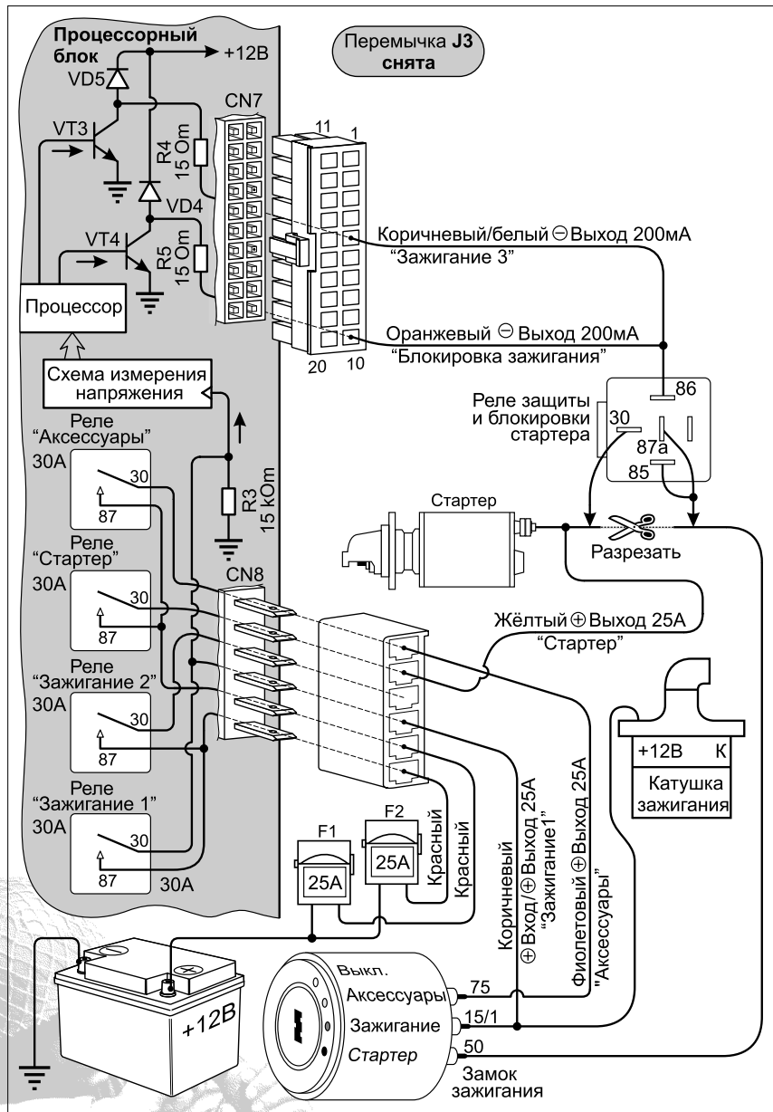
Рис. 20. Схема подключения нормально замкнутого реле блокировки и защиты стартера.
