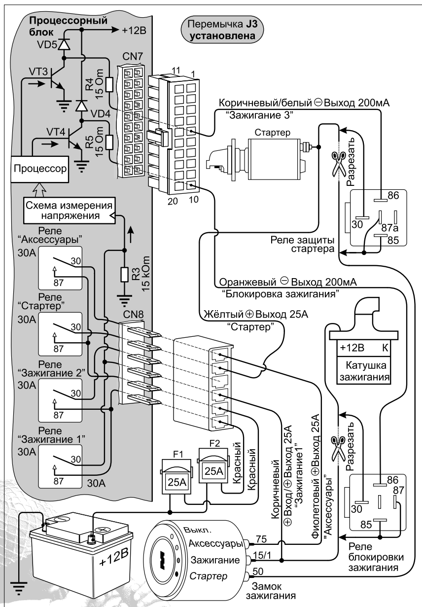
Рис. 18. Схема подключения нормально разомкнутого реле блокировки зажигания и реле защиты стартера.
