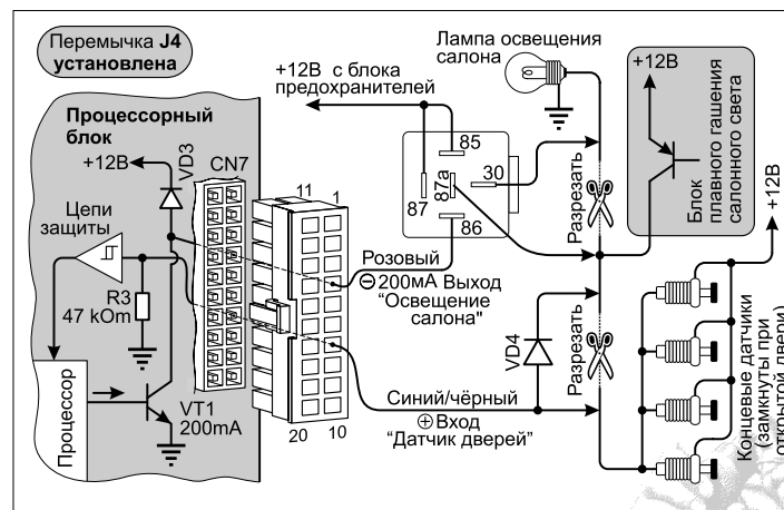
Рис.13. Подключение входа датчиков дверей и выхода управления освещением салона. Для автомобилей, в которых включение освещения салона производится при подаче +12В. Быстрое гашение освещения салона после того, как он был включен системой PARTISAN RX-5.
