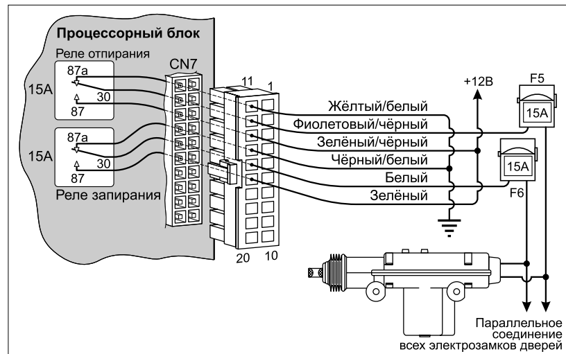
Рис. 5. Схема подключения к ЦЗ автомобиля с управлением положительными импульсами – управление переключением между массой и +12В по двум линиям.
